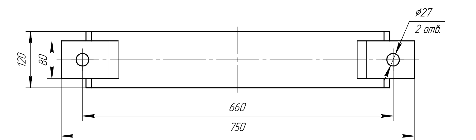
Дет. поз. 2 (1:5)
