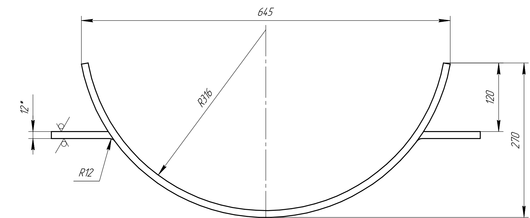
Дет. поз. 3
