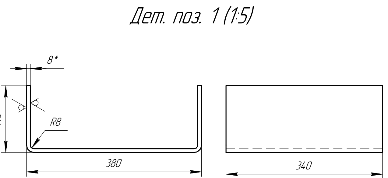
Дет. поз. 1 (1:5)
