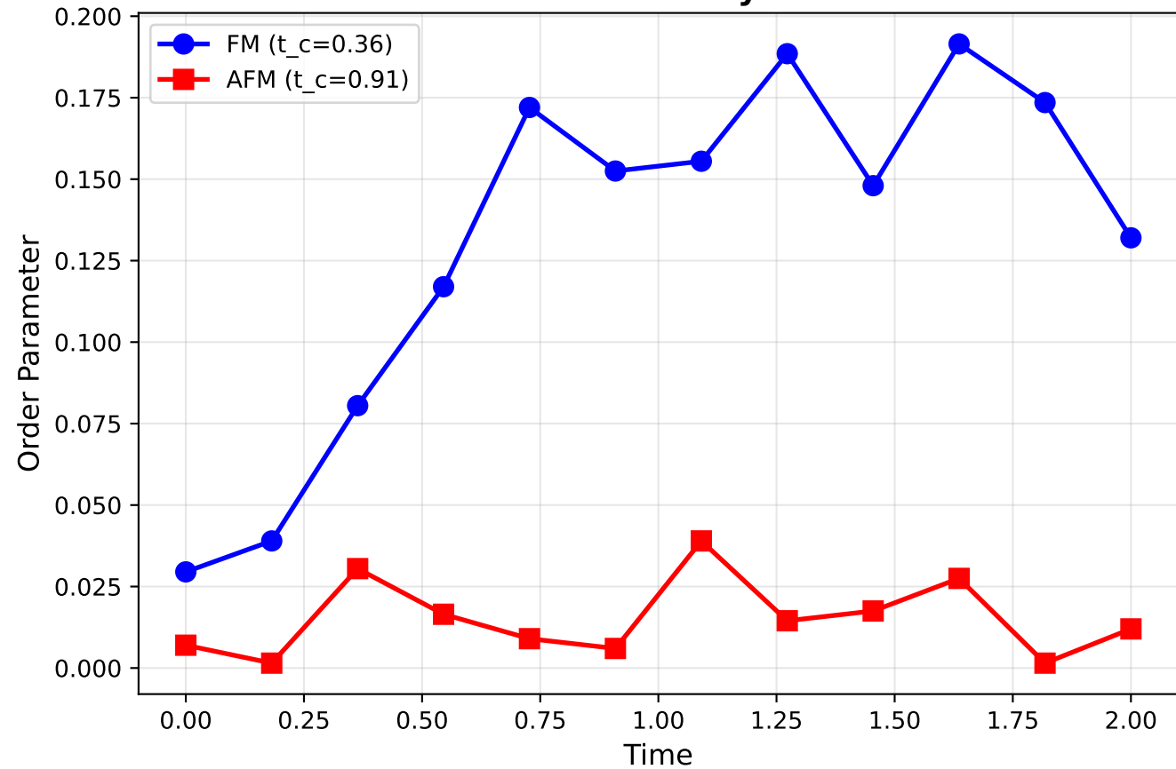
E2: FM vs AFM Dynamics
