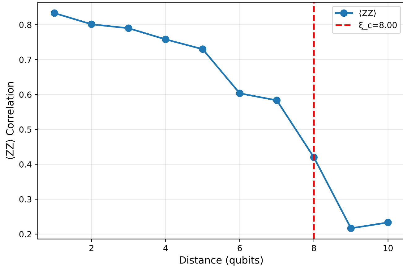
E1: Spin Correlation Decay
