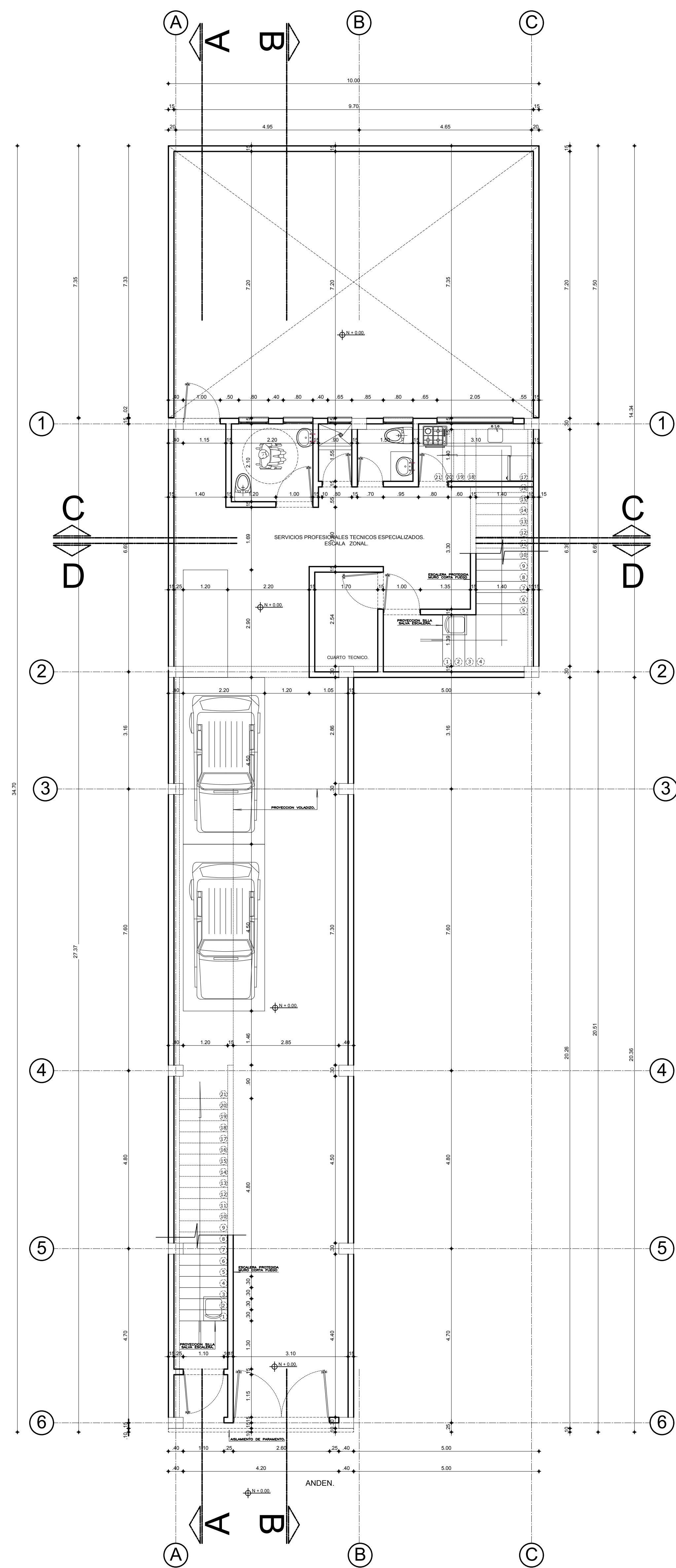
PLANTA PISO 1. ESCALA : 1 : 50.
