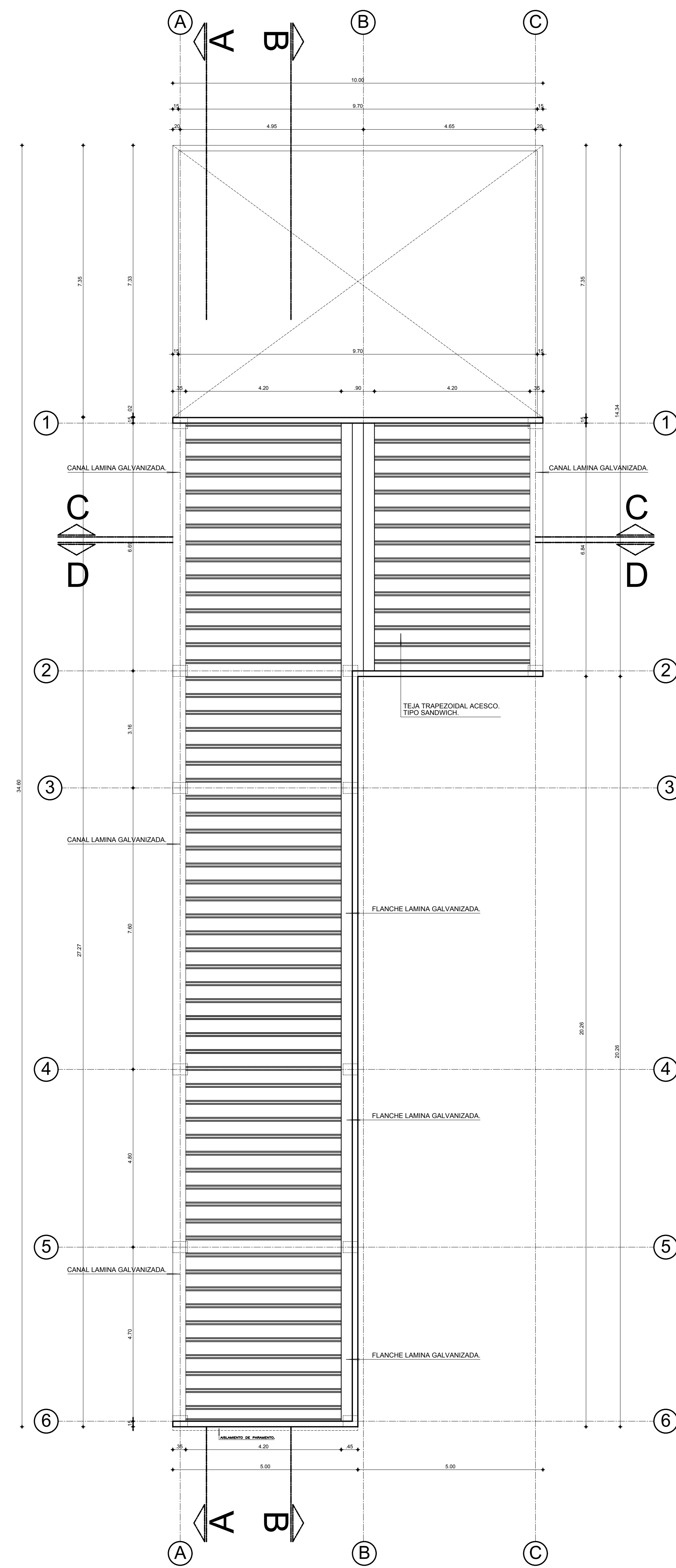
PLANTA DE CUBIERTAS. ESCALA : 1 : 50.
