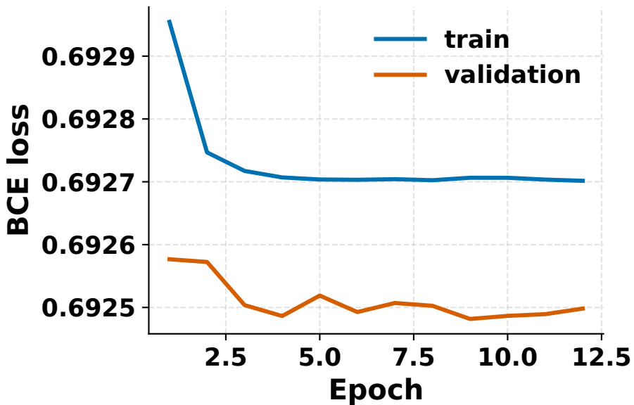
DNN-Aseeri — loss
