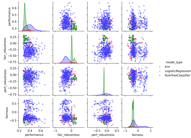
Figure 6: La figura mostra il RS inter-family che si divide nei gruppi delle tre famiglie osservate.
