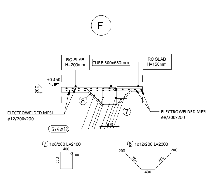
SECTION D-D 1:50
