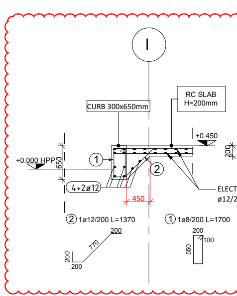
SECTION A-A 1:50
