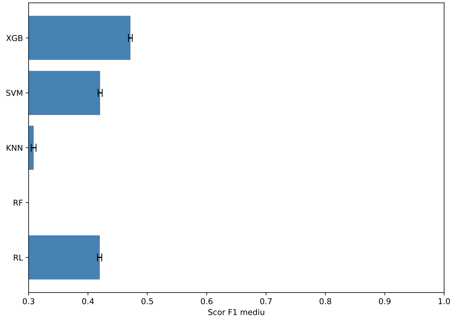
Scor F1 mediu(varianta normala) +- deviatie
