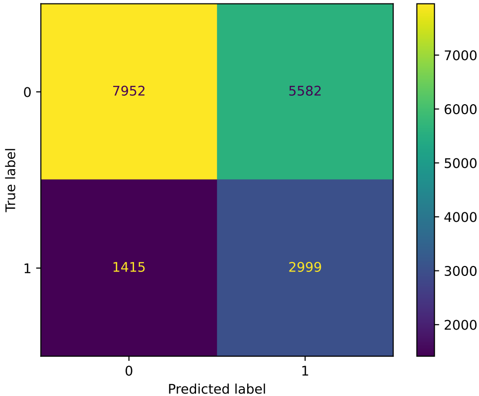
Matrice de confuzie - Random Forest
