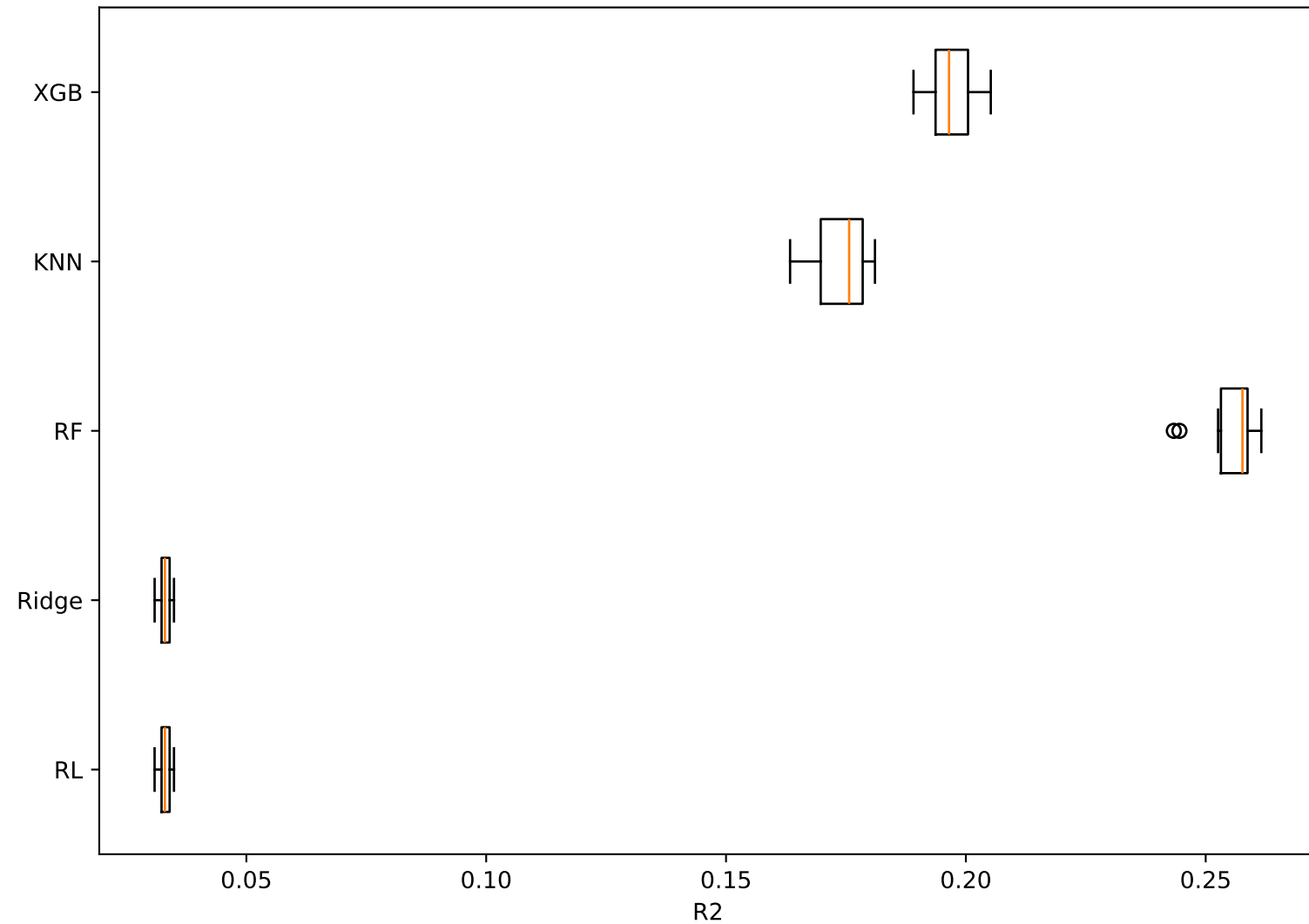
Distributia R2(varianta optimizata) pe 10 rulari
