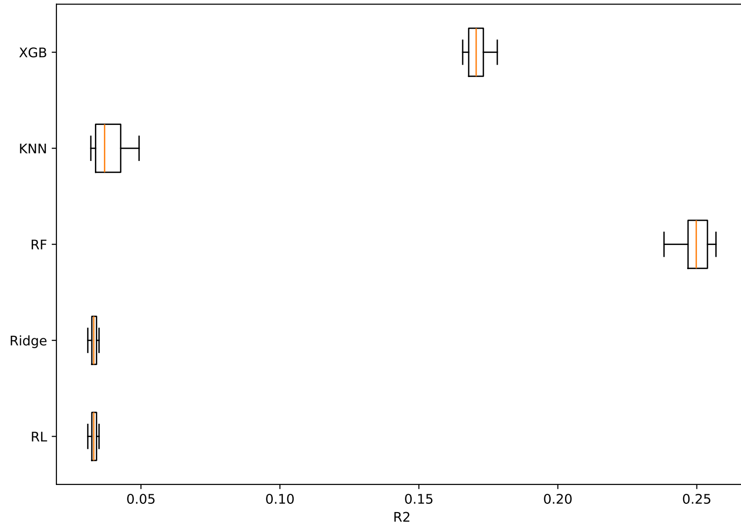
Distributia R2(varianta normala) pe 10 rulari
