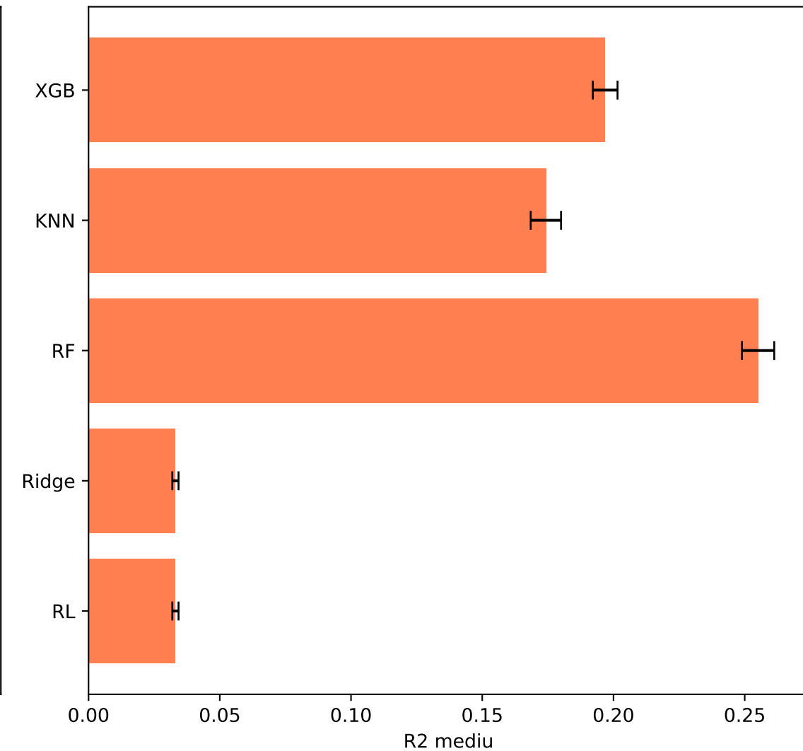
R2 mediu +/- deviatie(10 rulari)
