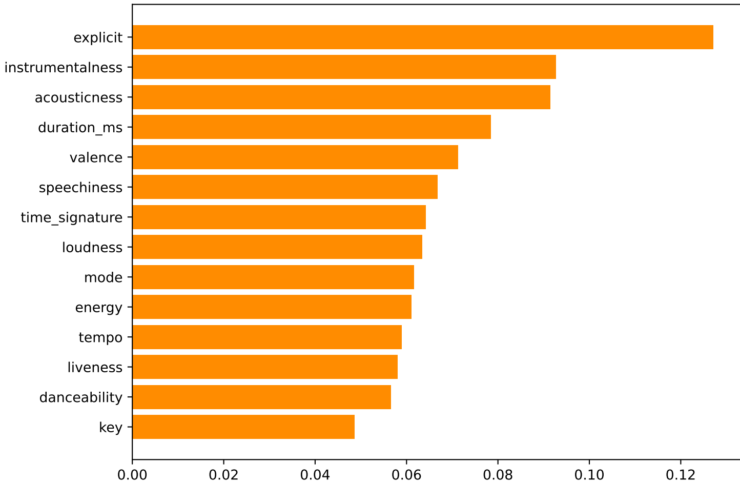
Importanta caracteristicilor - XGBoost regresie
