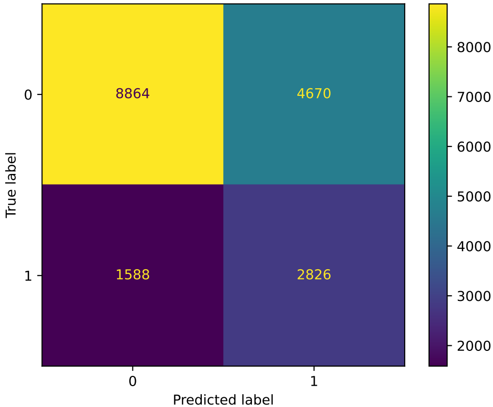
Matrice de confuzie - XGBoost
