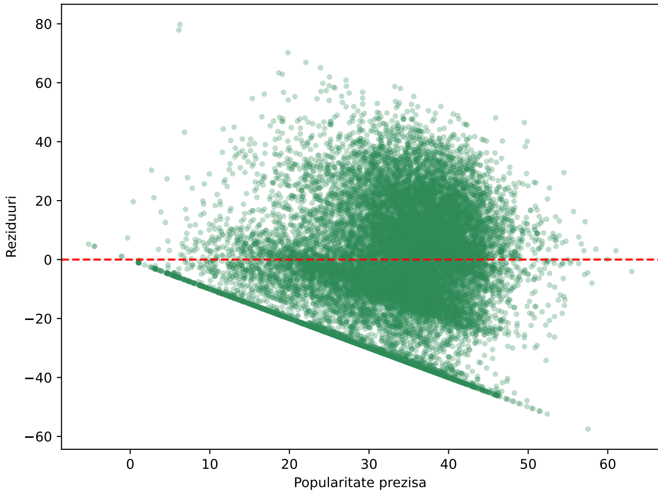
Grafic reziduuri-XGBoost
