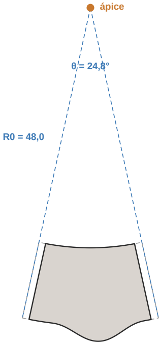
gris discontinuo: sector completo · relleno: base con hueco de cierre y pico (hacia abajo en este esquema)
