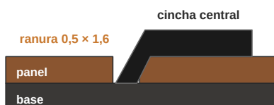
Ranura del panel (corte)
