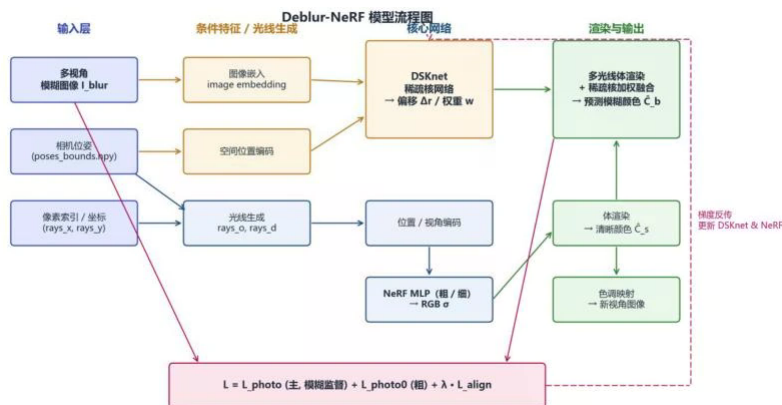
图3-3 Deblur-NeRF 模糊建模数据流程
