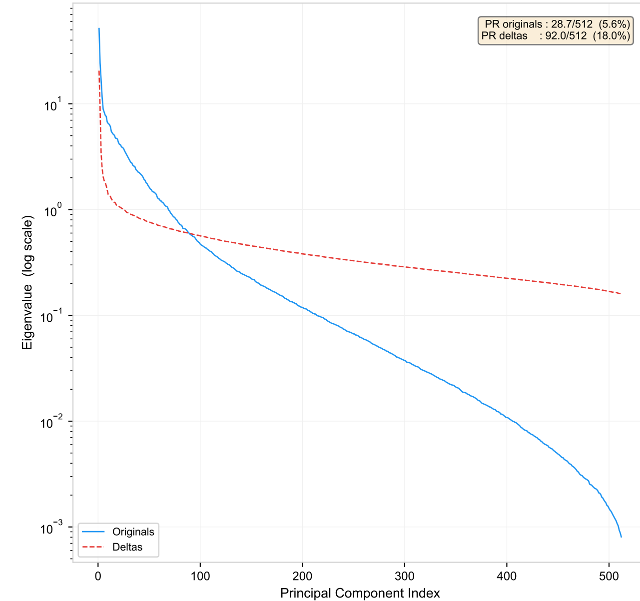
C) Eigenvalue Spectrum
