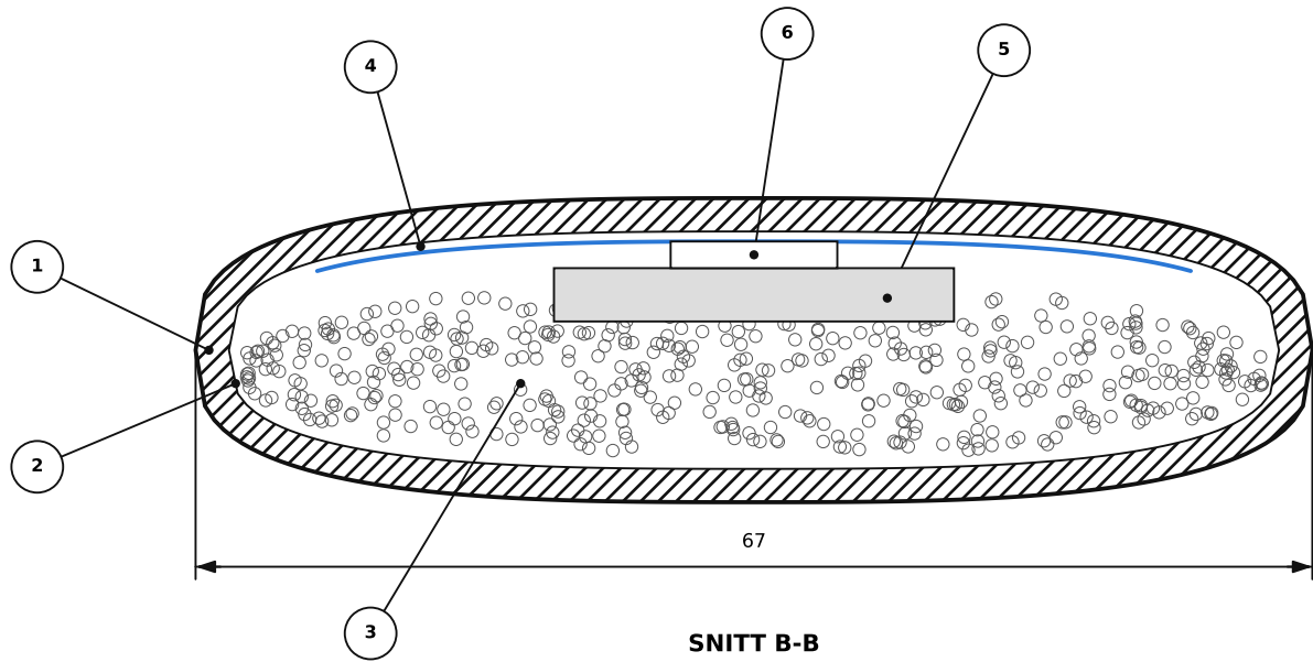
SNITT B-B
