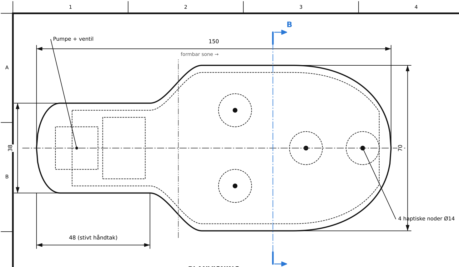
PLANVISNING
