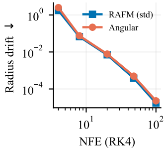
Student- t d16
