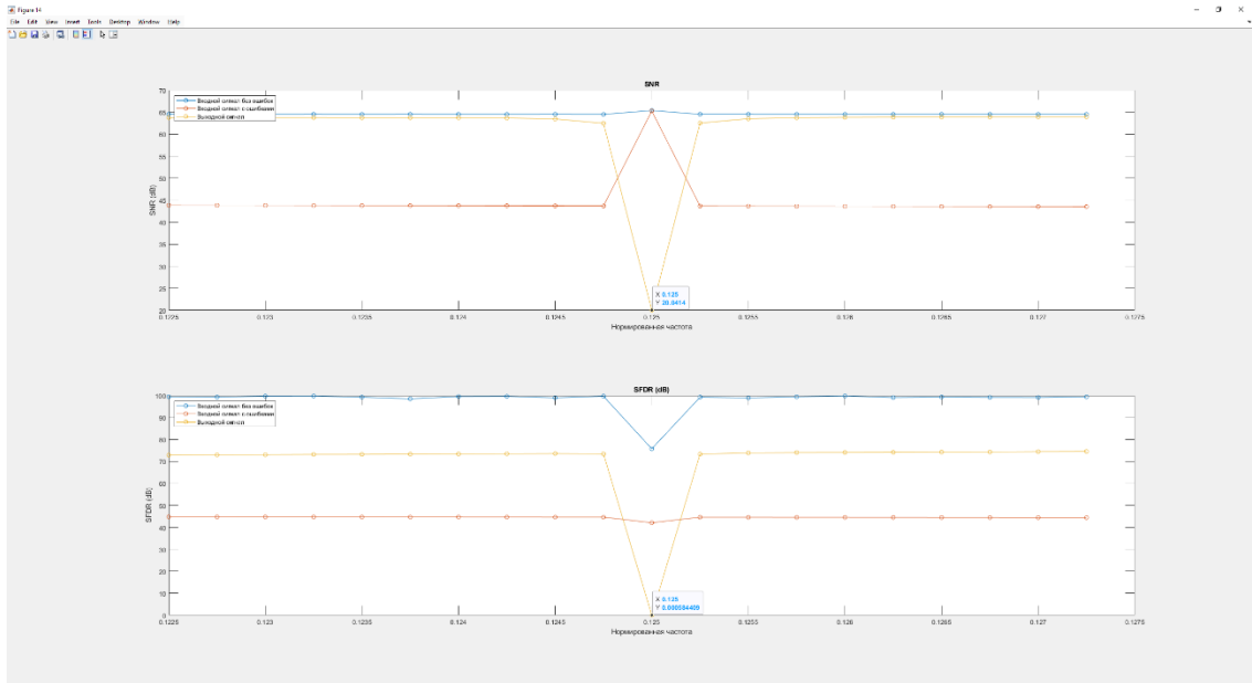
Рисунок 10. Моделирование возле границы зоны Найквиста с шагом входного сигнала 1 МГц, при \Delta_1 = 0.01 T_s , \Delta_2 = 0.03 T_s , \Delta_3 = 0.02 T_s , \Delta_4 = 0.01 T_s .
