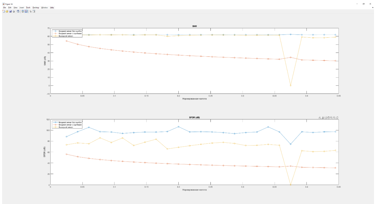
Рисунок 11. Результаты моделирования при N = 12\text{bit} , M = 4 , F_s = 4\text{ ГГц} , F_c = 1\text{ ГГц} , \Delta_1 = 0.01 T_s , \Delta_2 = 0.06 T_s , \Delta_3 = 0.03 T_s , \Delta_4 = 0.05 T_s .
