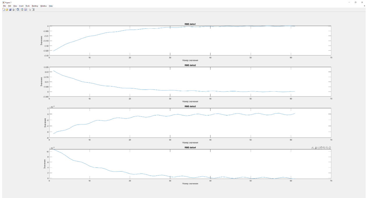
Рисунок 10. График RMS значений time skew для M=4 . Сходимость около 30 циклов [1] стр.12
