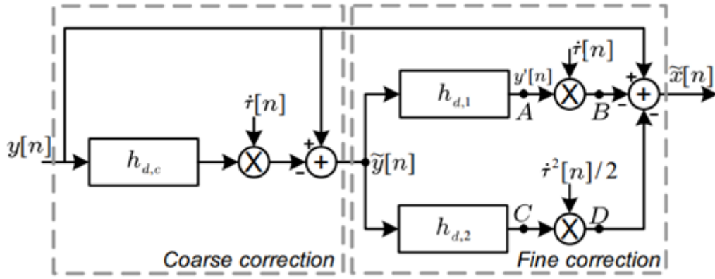
Рисунок 6. Схема коррекции time skew.
