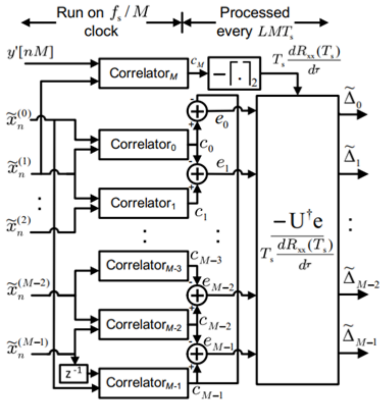
Рисунок 5. Схема оценки time skew
