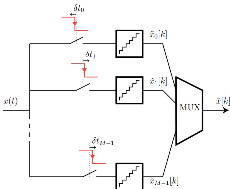
Рисунок 1. Схема TI-ADC
