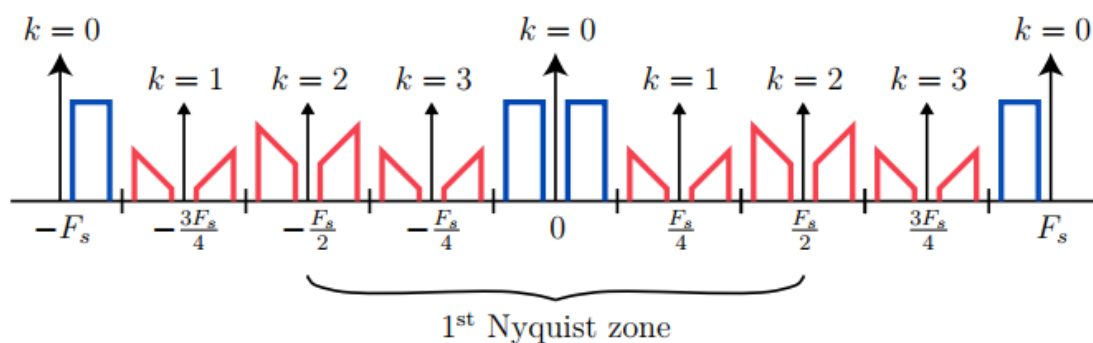
Рисунок 2. Спектр выходного сигнала АЦП рассогласованного во времени
