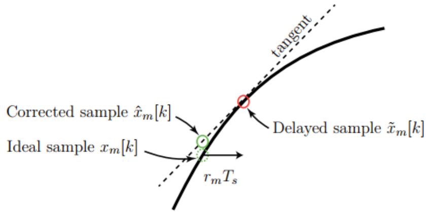
Рисунок 3. Коррекция time skew
