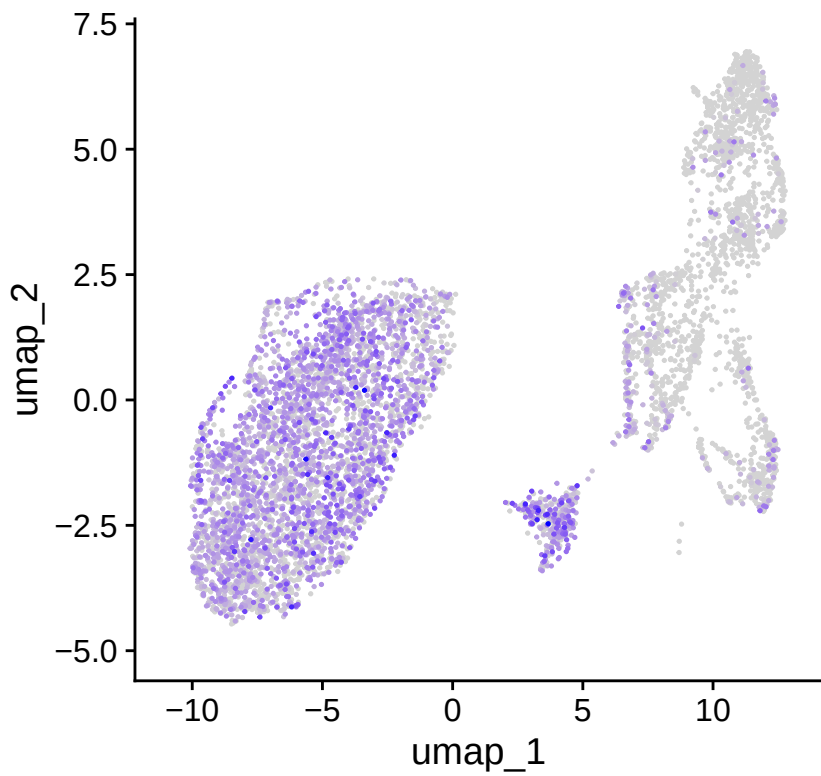
Gad2
