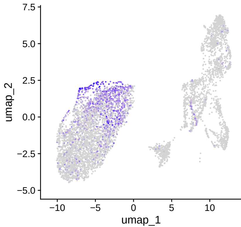
Fabp7
