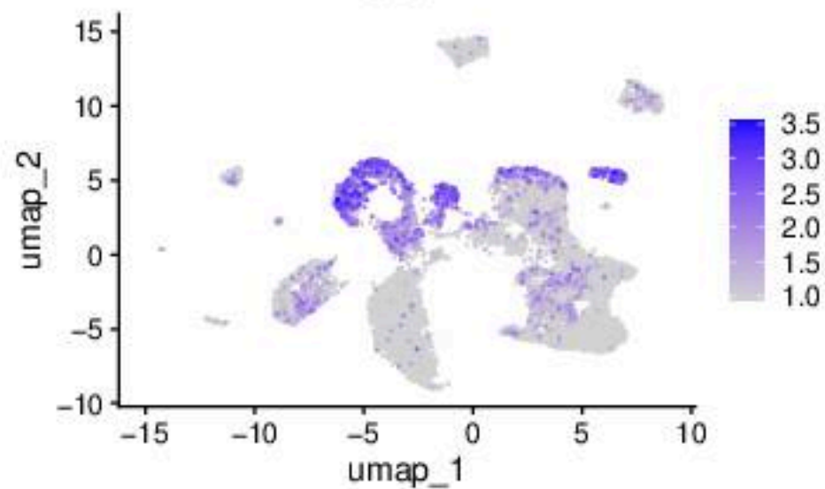
Aldh1l1
