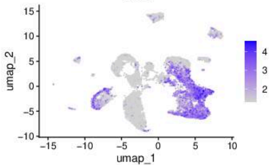
Hes5
