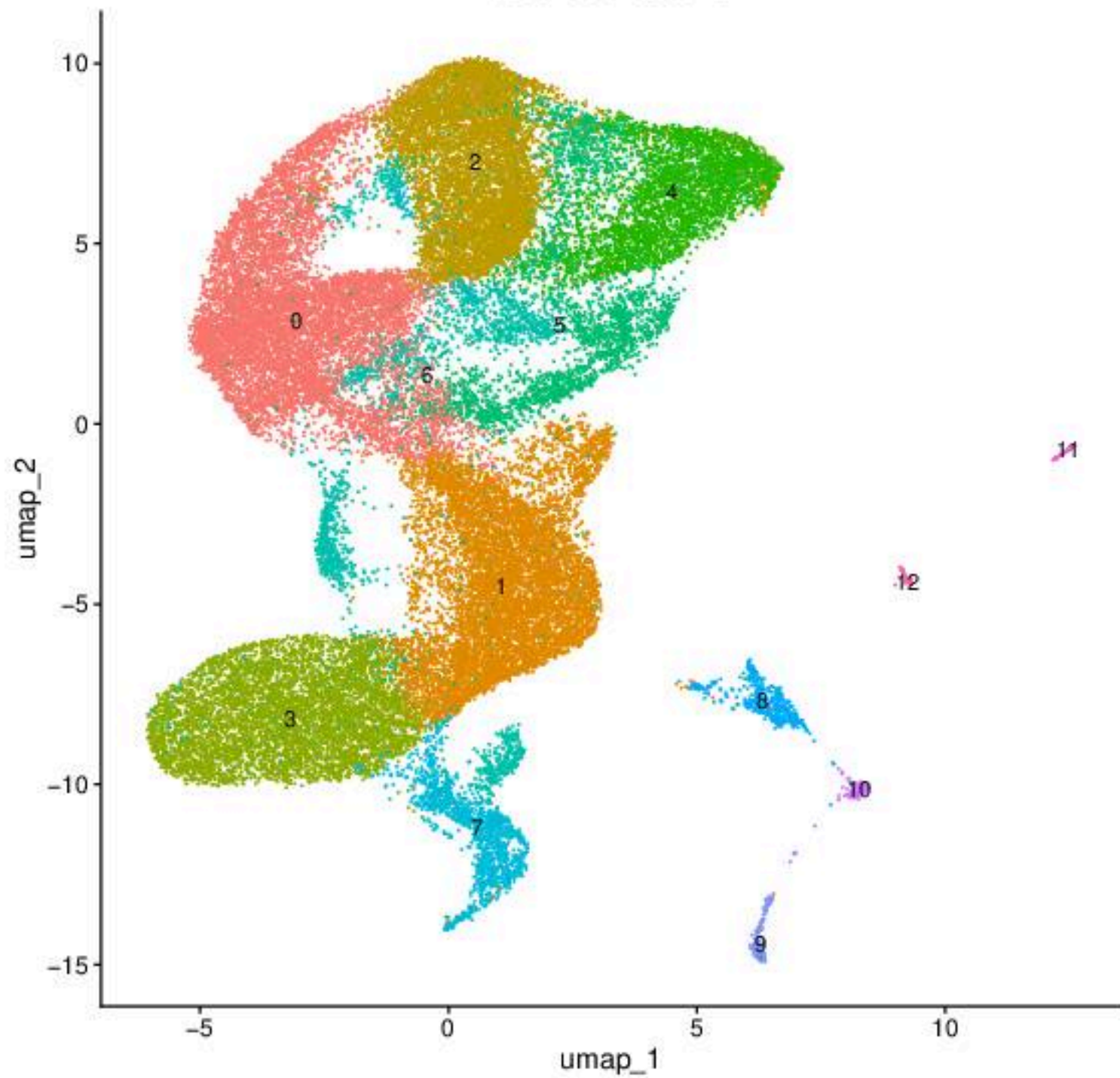
Seurat clusters
