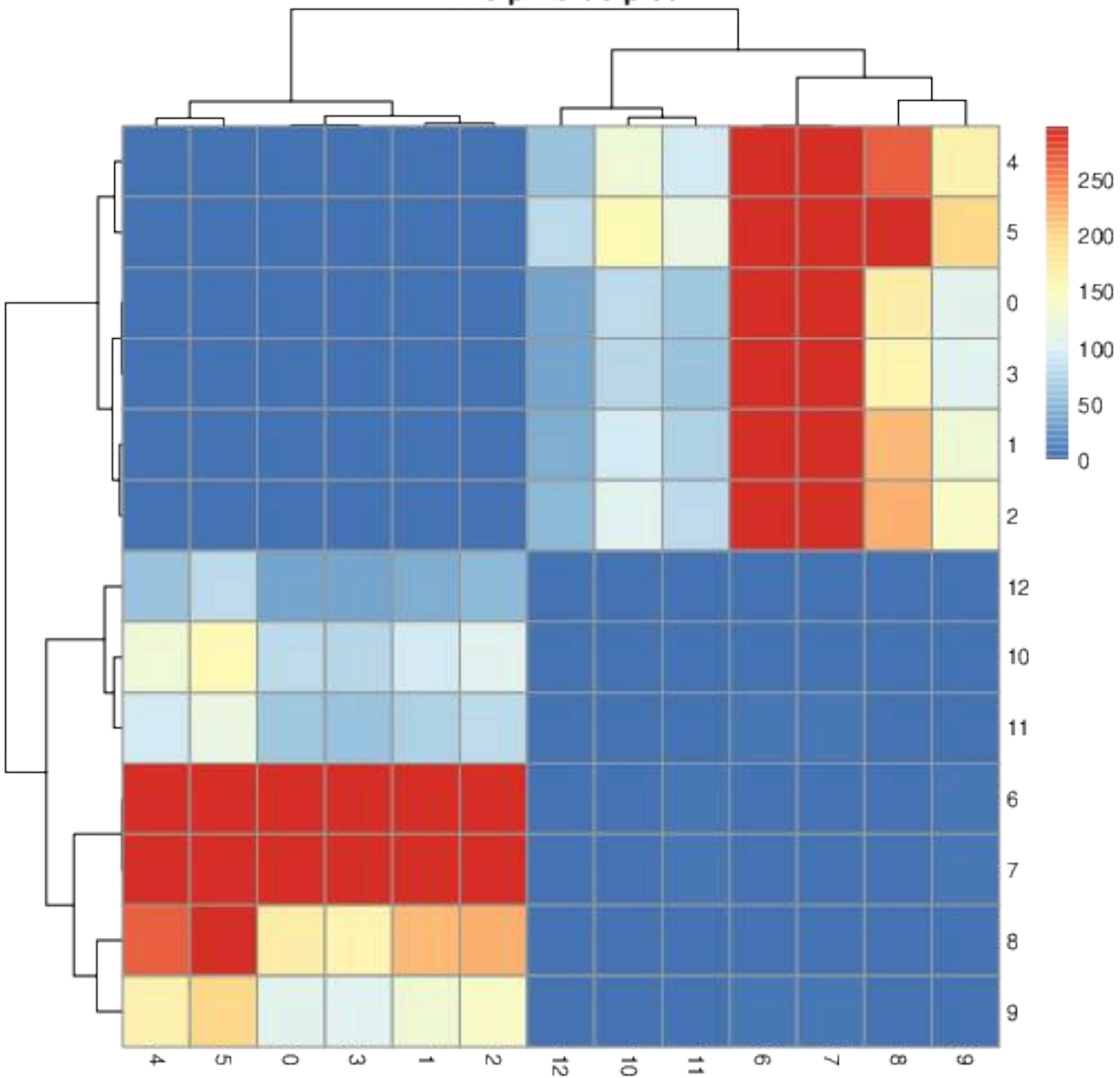
D13 p-value plot
