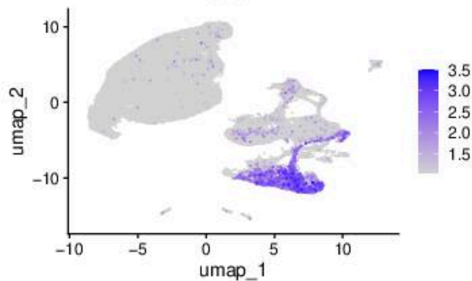
Aldh1l1
