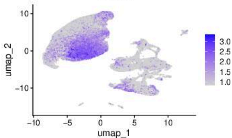
Hes5
