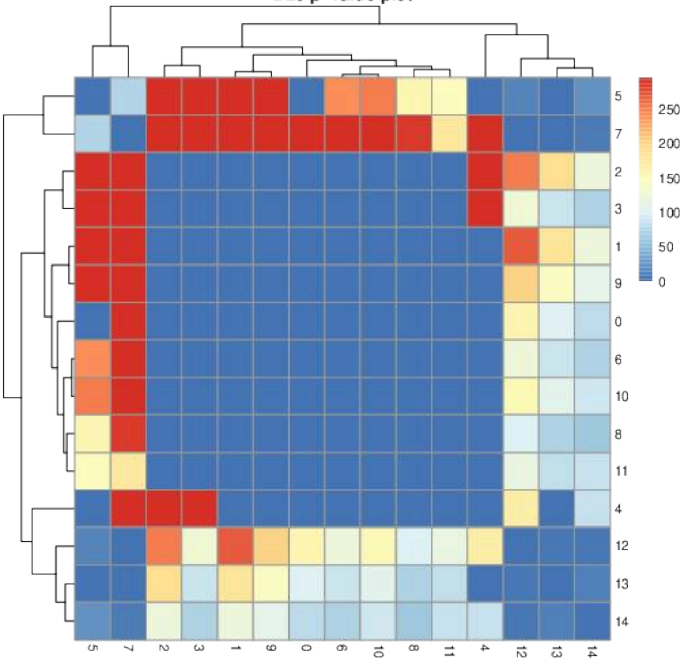
D20 p-value plot
