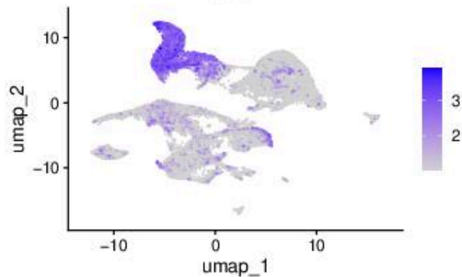
Aldh1l1
