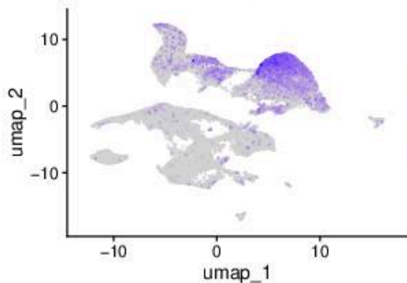
Hes5
