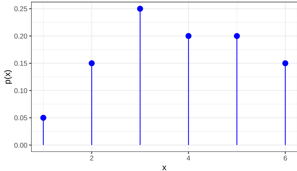
Função de Probabilidade de X
