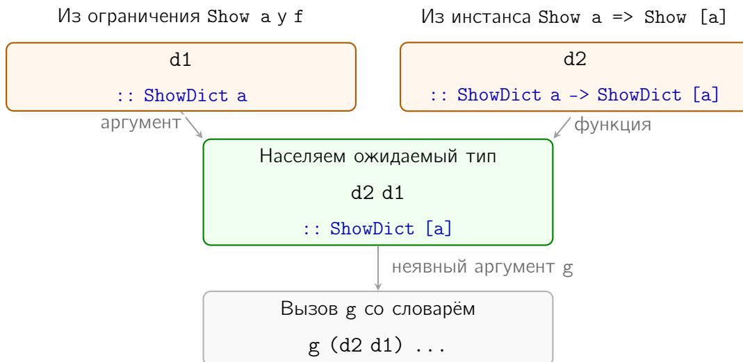
Рис. 12: Население типа словаря: компилятор находит терм d2 d1 типа ShowDict [a] и подставляет его в вызов g (вызов со словарём показан схематично).
