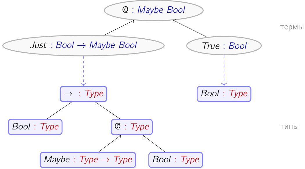
Рис. 5: Два этажа типизации выражения \text{Just True} . Вершинам дерева терма приписаны типы (синим). Каждый тип сам является деревом (пунктирные стрелки), и его вершинам приписаны кайнды (красным).
