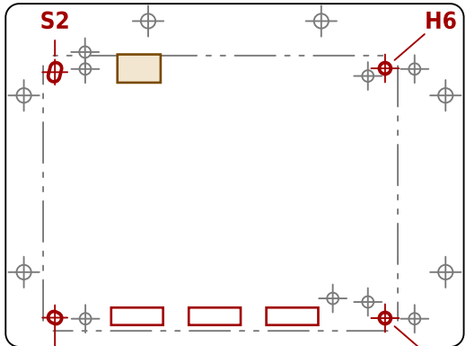
TT04-05 (TT04, TT05) board rev v1.2.2, v1.2.3 offset X 11.05 Y 4.72 mm
