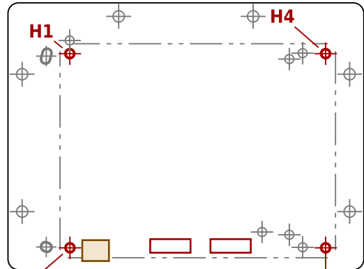
TT01-03 (TT01, TT02, TT03) board rev tt123-v2.2.6 offset X 19.76 Y 4.54 mm
