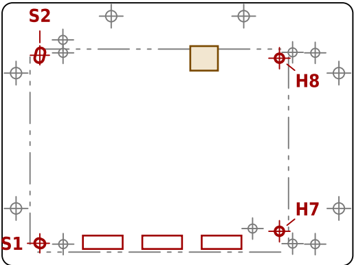
TT06-08 (TT06, TT07, TT08) board rev v2.0.1, v2.1.0, v2.1.2 offset X 10.74 Y 5.22 mm
