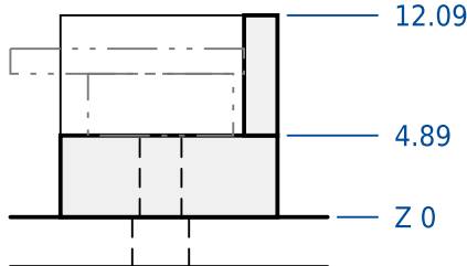
SECTION B-B, 2:1
