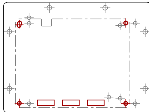
TT04-05 (TT04, TT05) board rev v1.2.2 offset X 11.05 Y 4.72 mm
