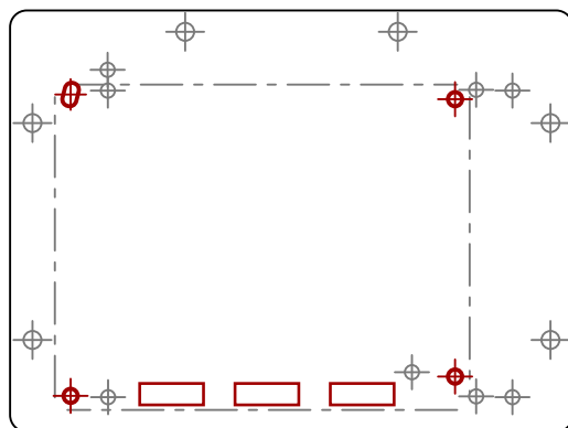
TT06-08 (TT06, TT07, TT08) board rev v2.0.1 offset X 10.74 Y 5.22 mm
