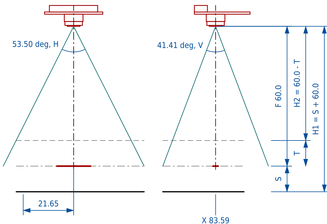
PLAN, 1:2
