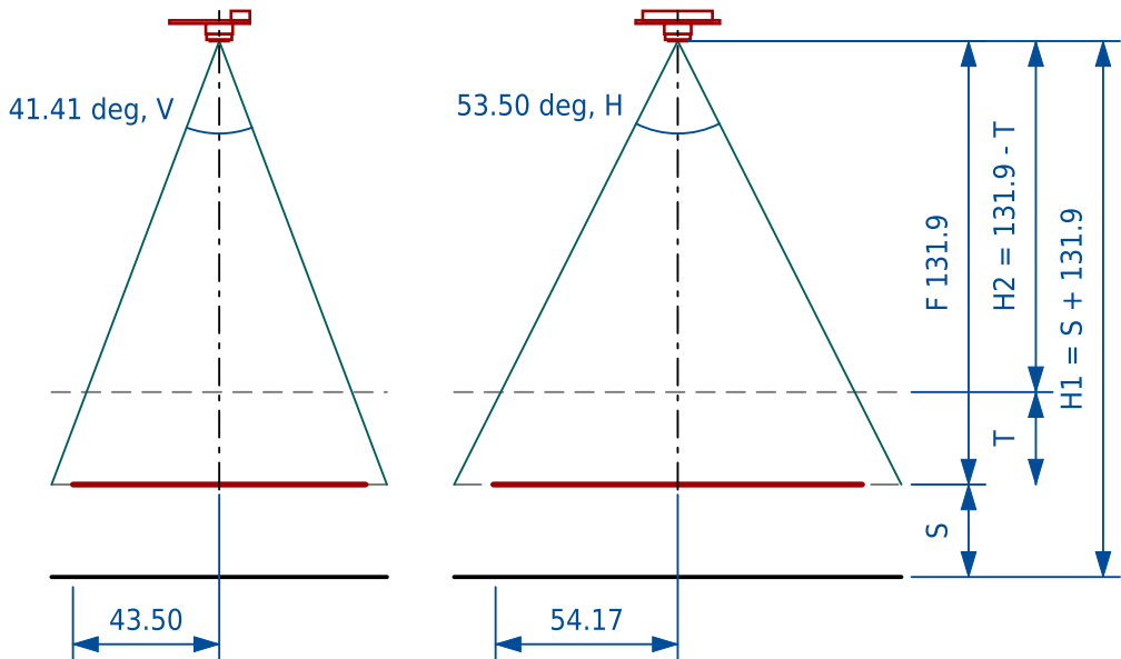
PLAN, 1:5
