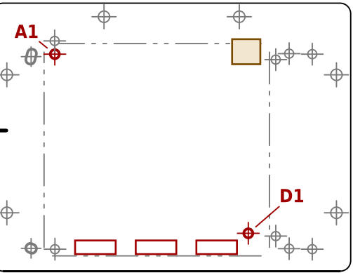
DB ETR v3.2 TT09, TTSKY25a, TTSKY25b, TTGF0p2 board rev v3.2
