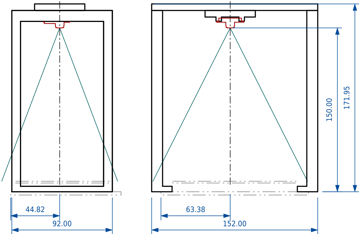
END ELEVATION
