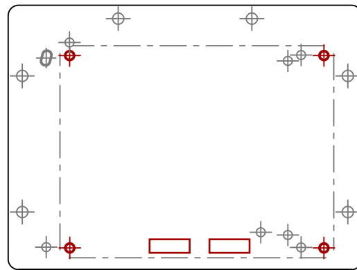
TT01-03 (TT01, TT02, TT03) board rev tt123-v2.2.6 offset X 19.760 Y 4.535
