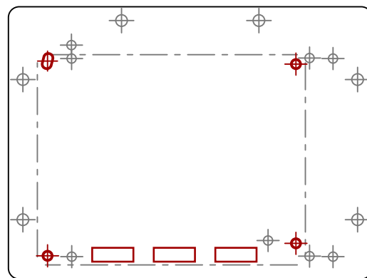
TT06-08 (TT06, TT07, TT08) board rev v2.0.1 offset X 10.745 Y 5.225
