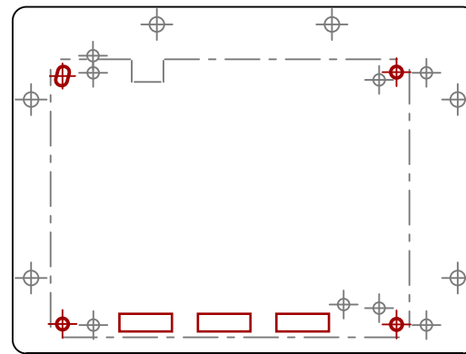
TT04-05 (TT04, TT05) board rev v1.2.2 offset X 11.055 Y 4.725
