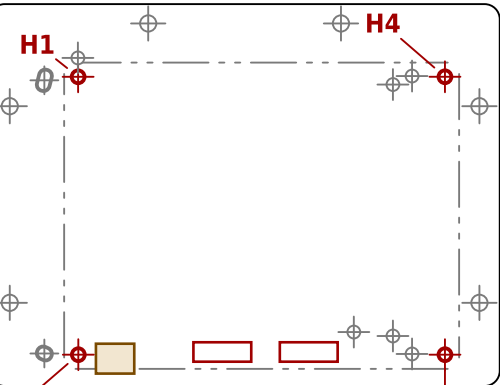
TT01-03 (TT01, TT02, TT03) board rev tt123-v2.2.6 offset X 19.76 Y 4.54 mm
