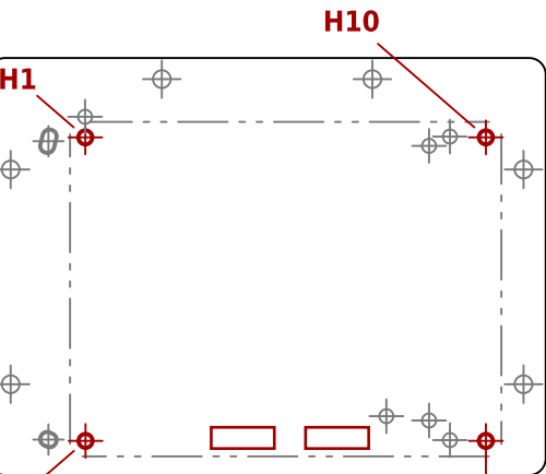
TT01-03 (TT01, TT02, TT03) board rev tt123-v2.2.6 offset X 19.76 Y 4.54 mm
