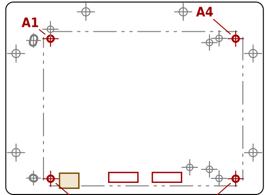
DB mpw TT02, TT03 board rev tt123-v2.2.5, tt123-v2.2.6
