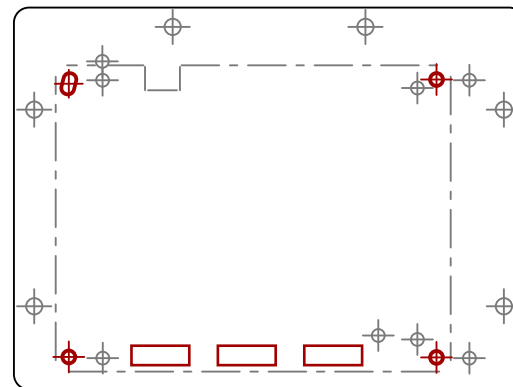
TT04-05 (TT04, TT05) board rev v1.2.2 offset X 11.055 Y 4.725
