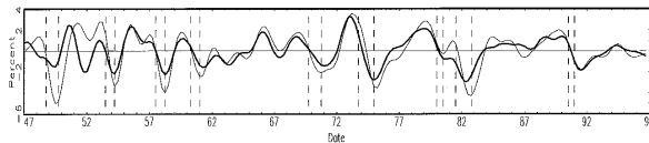
Fig. 3.9. Consumption (total).
