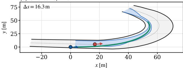
(d) Pass, t=28.9\text{ s}
