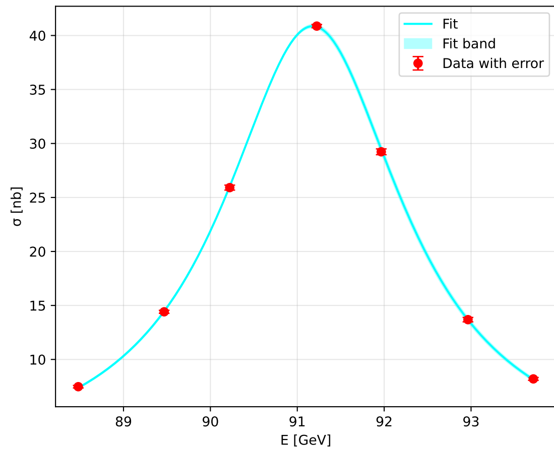
e^+e^- \rightarrow \text{hadronisch}
