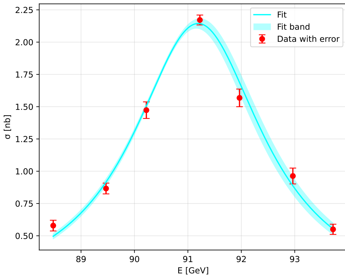
e^+e^- \rightarrow \tau^+\tau^-
