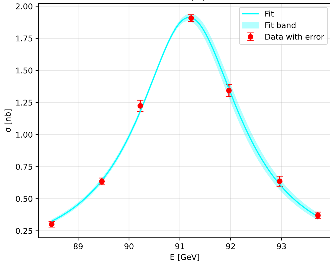
e^+e^- \rightarrow \text{hadronisch}
