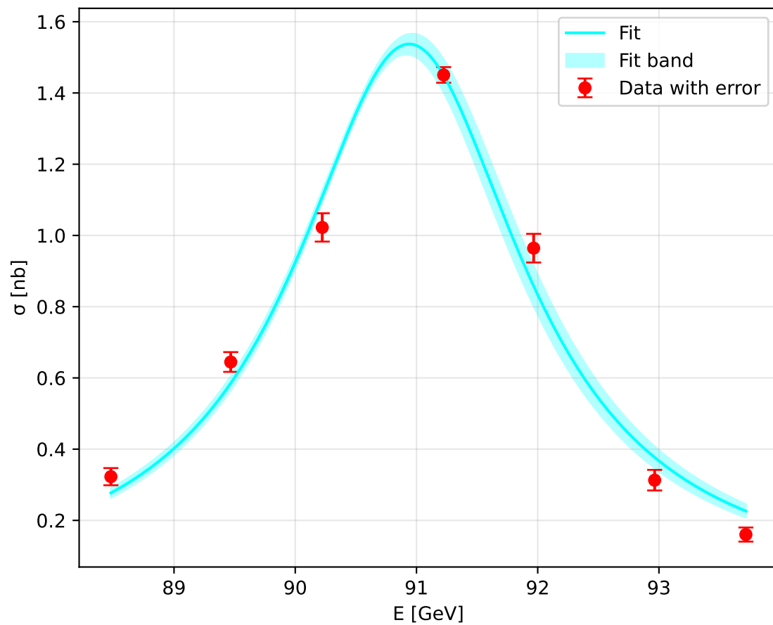
e^+e^- \rightarrow \tau^+\tau^-
