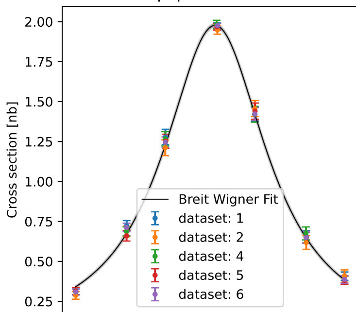
\mu^+\mu^- channel
