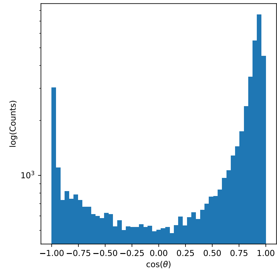
e + e - channel
