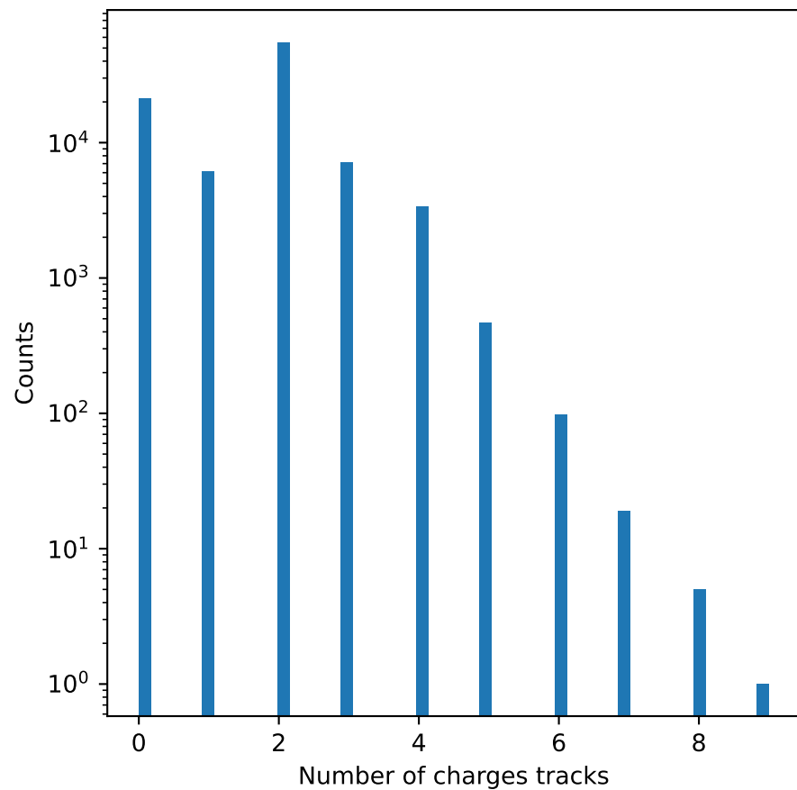
e + e - channel
