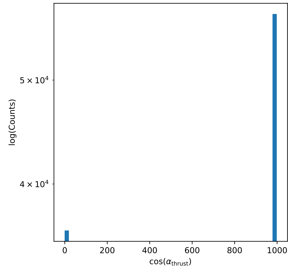
e + e - channel
