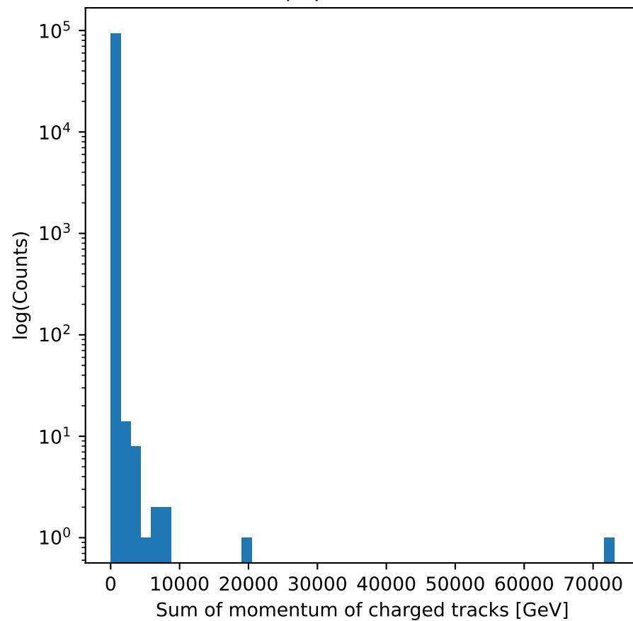
\mu^+\mu^- channel
