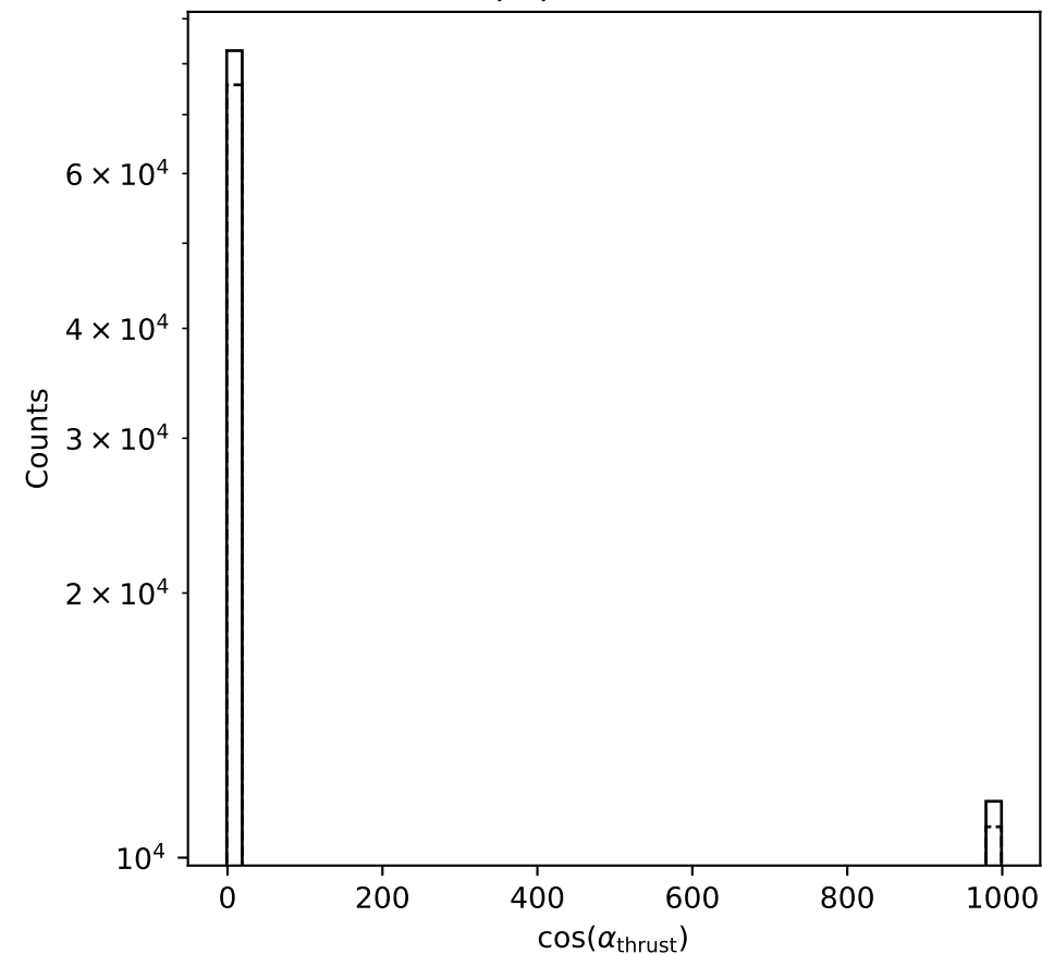
\mu^+\mu^- channel
