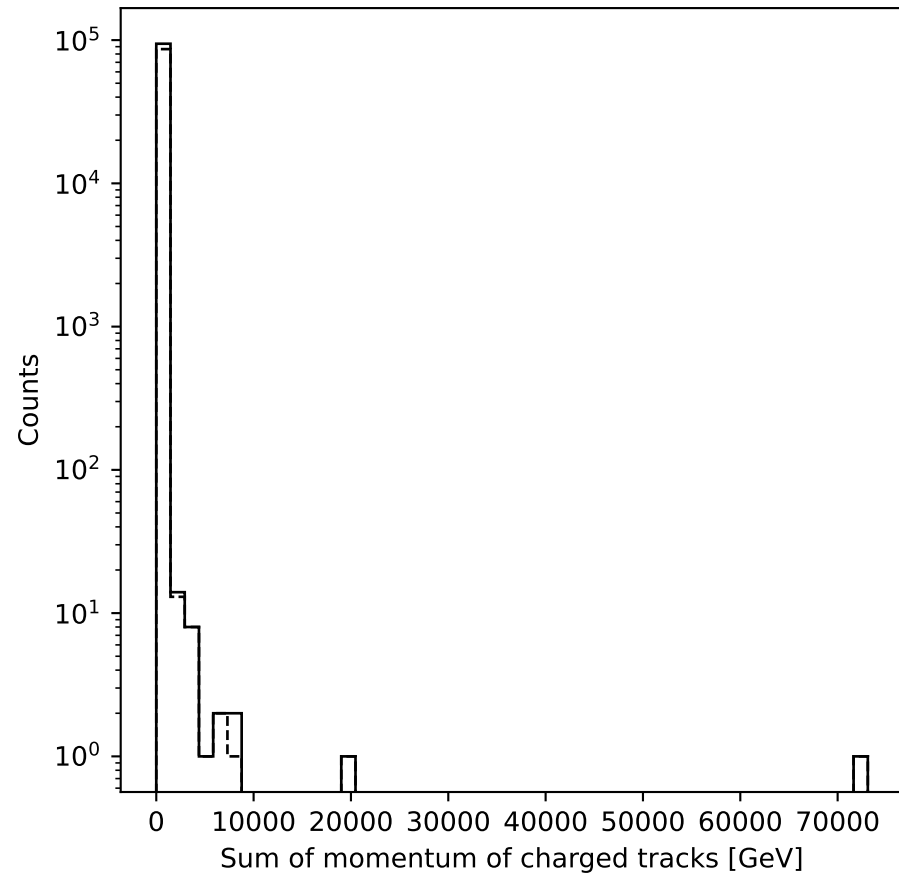
\mu^+\mu^- channel
