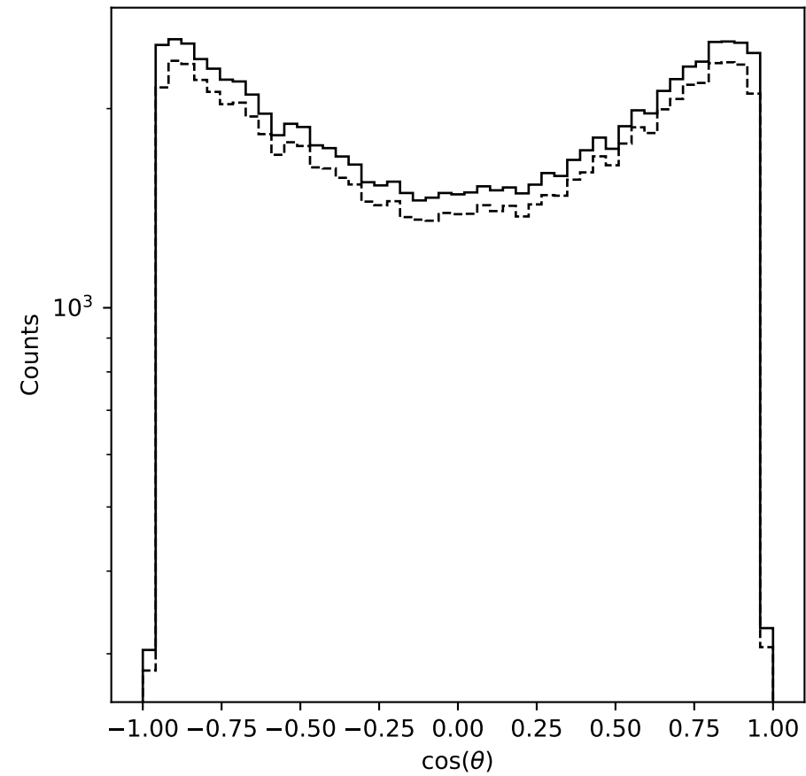
\mu^+\mu^- channel
