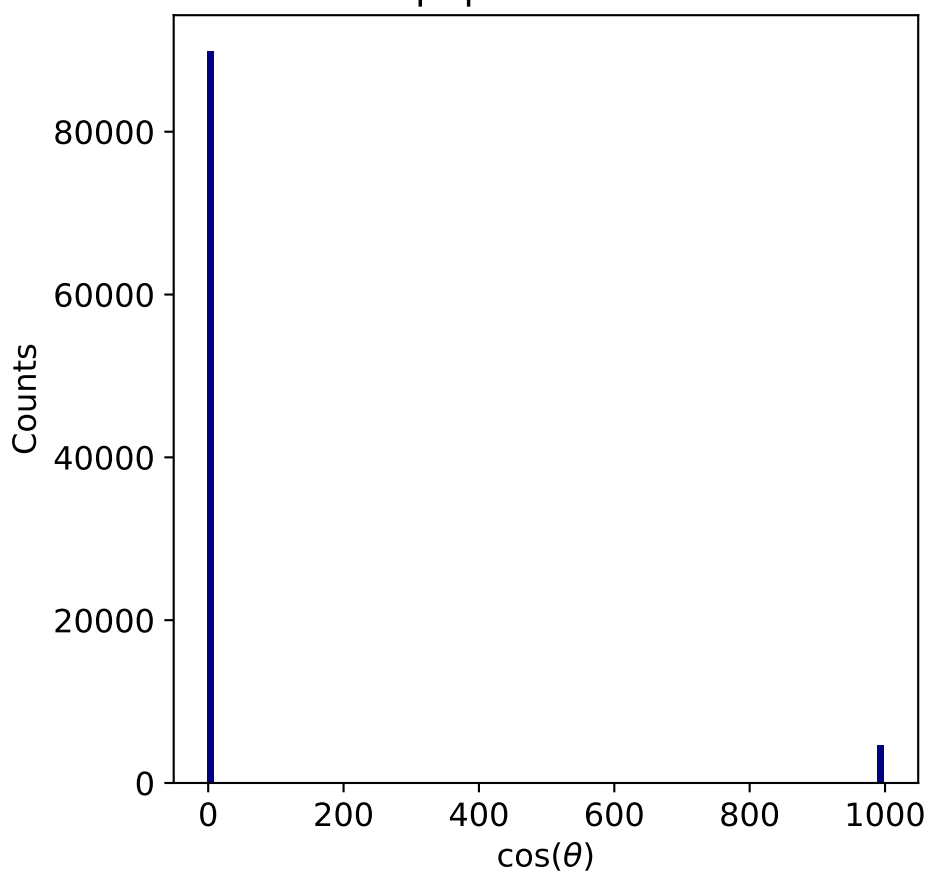
\mu^+\mu^- channel
