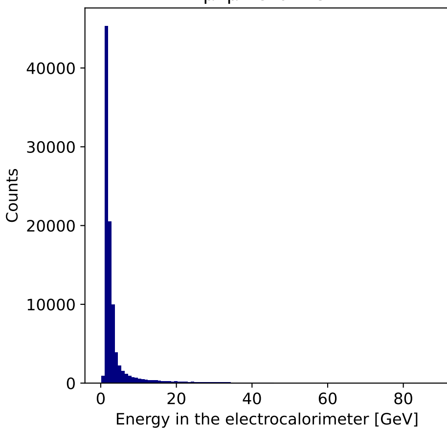
\mu^+\mu^- channel
