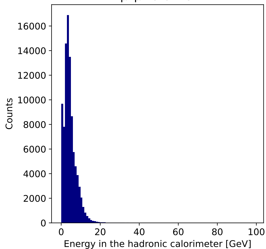
\mu^+\mu^- channel
