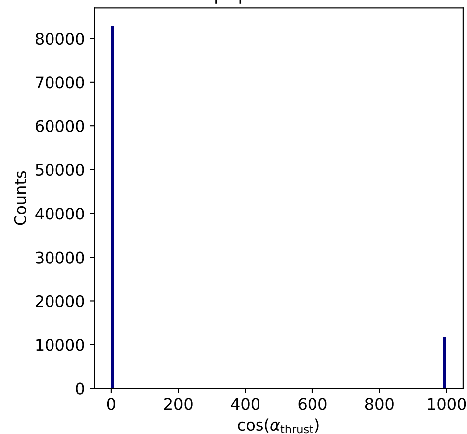
\mu^+\mu^- channel
