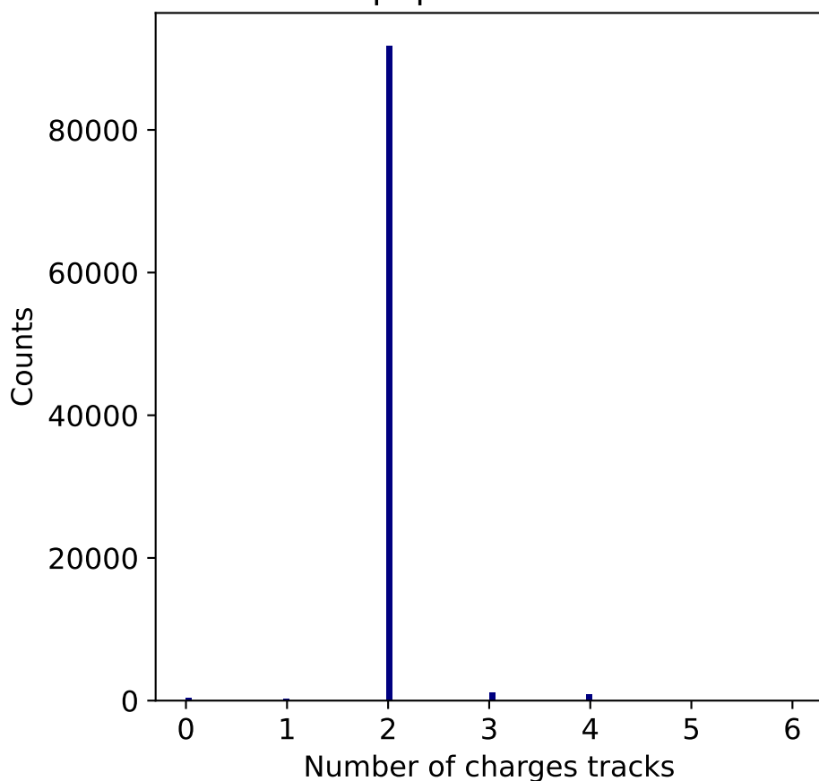
\mu^+\mu^- channel
