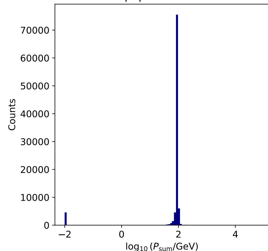
\mu^+\mu^- channel
