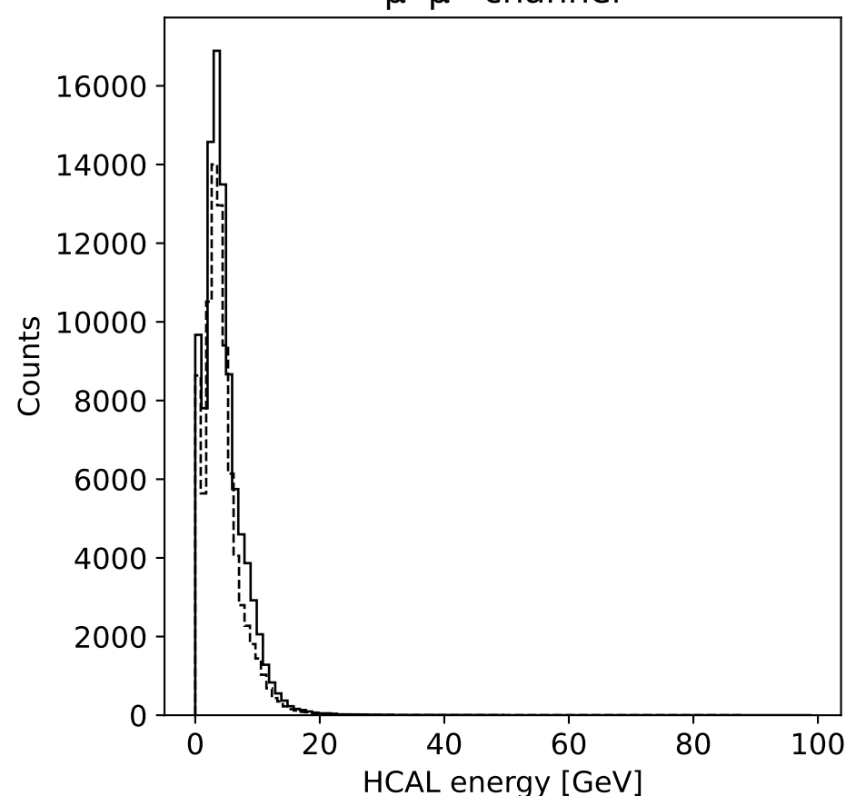
\mu^+\mu^- channel
