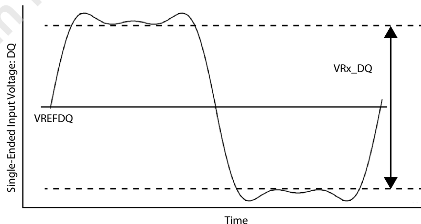
Figure 226 — VRx_DQ
